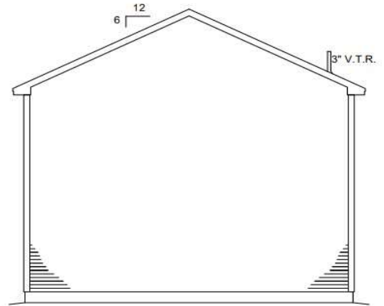
RIGHT ELEVATION
