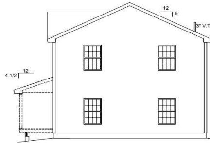
RIGHT ELEVATION
