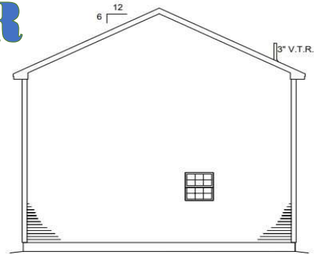
RIGHT ELEVATION
